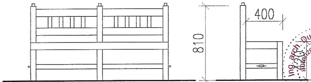
BOČNÝ POHĽAD
