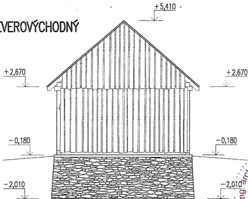
POHLAD JUHOVÝCHODNÝ
