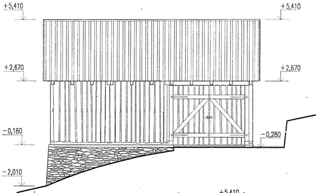
POHLAD SEVEROVÝCHODNÝ
